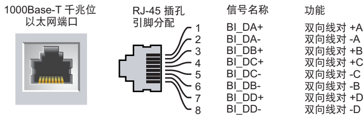
图 3 10/100/1000BASE-T 管理端口引出线
