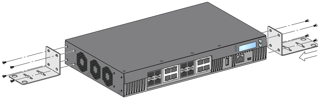
图 10 安装壁式安装托架
