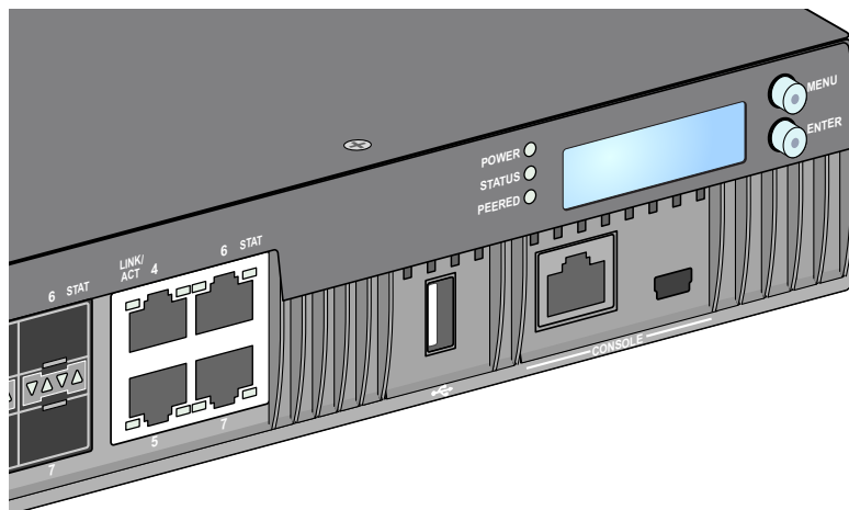
图 4 端口、LED 和 LCD 面板
