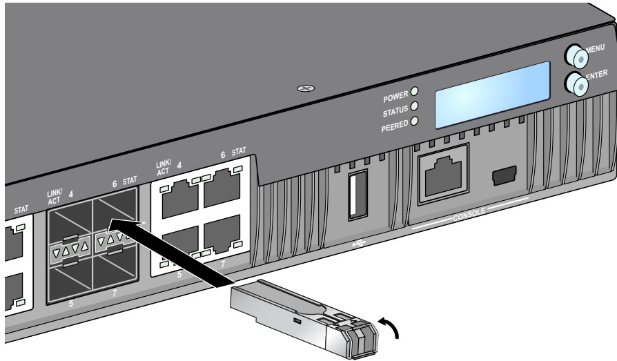
图 12 安装 SFP
