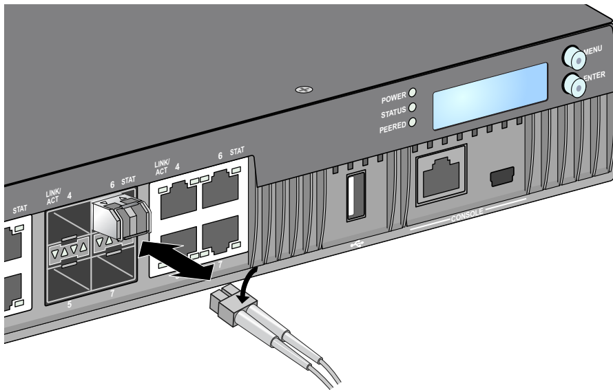
图 13 连接 LC 光纤电缆
