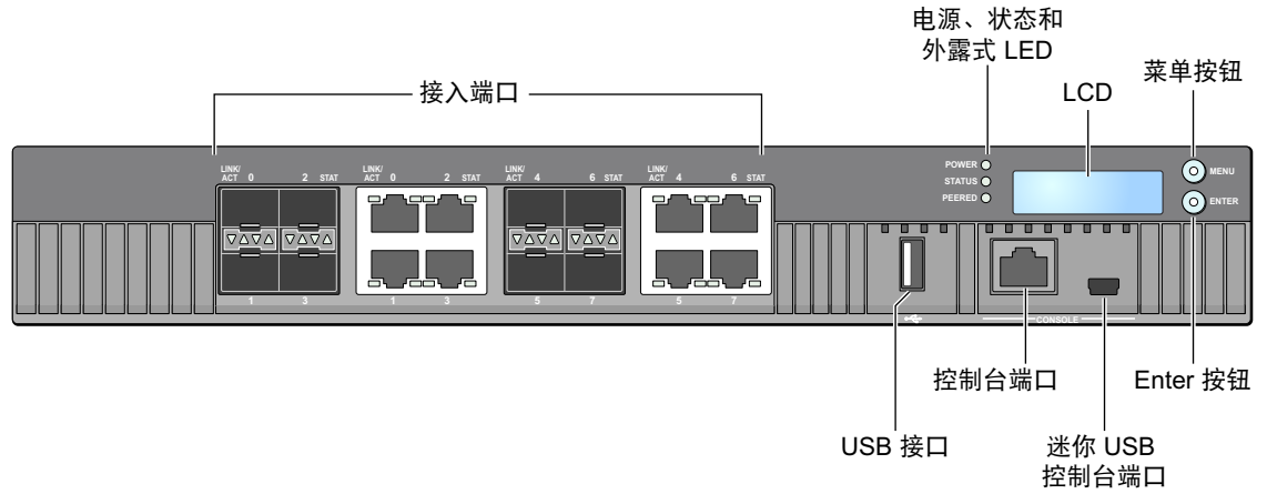
图 1 W-7030 控制器的前置面板
