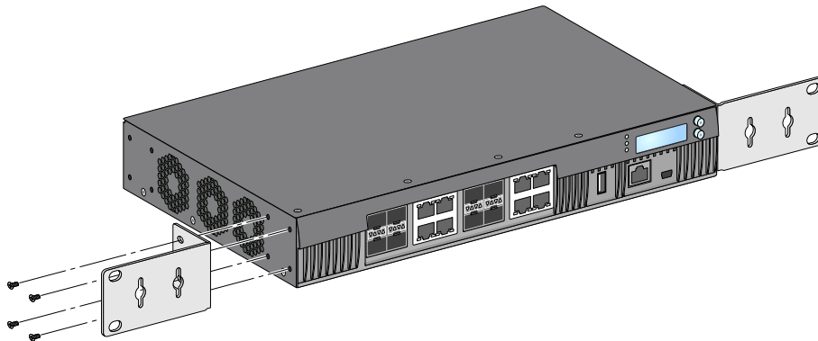
图 7 机架安装托架
